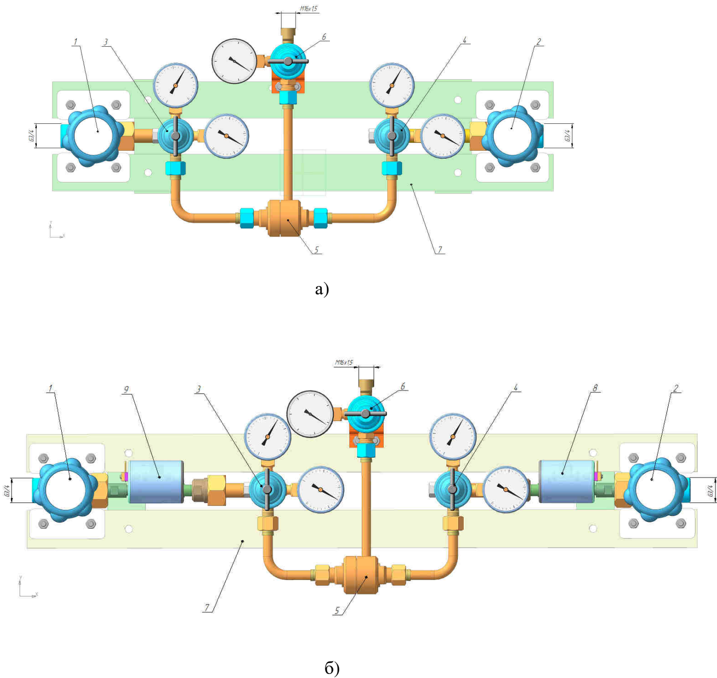
Рис.1 Щит автопереключения плеч перепускных газовых рамп.
